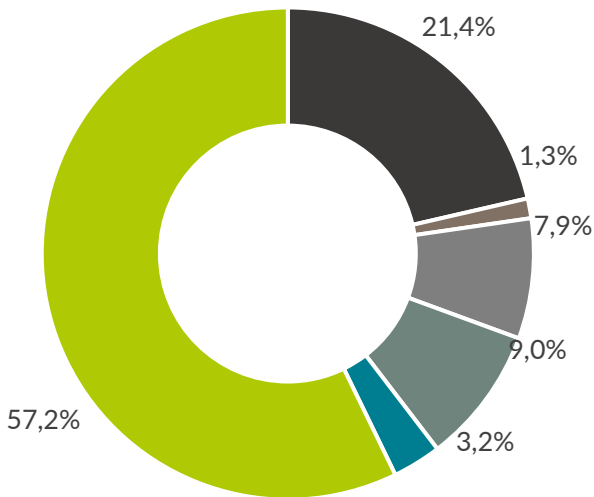
Verbleibender Energieträgermix
