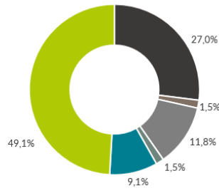
Verbleibender Energieträgermix
